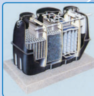
小型浄化槽
