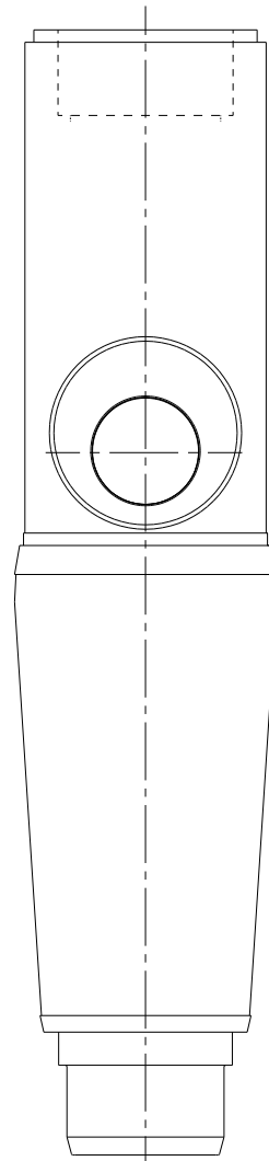
A矢視図
