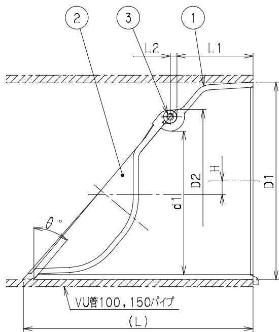
VU管：呼び径100, 150
