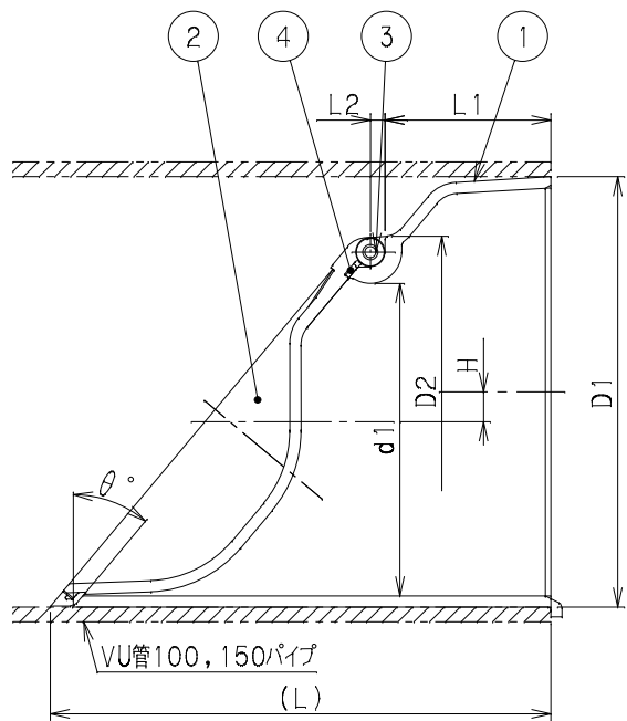
VU管：呼び径100, 150
