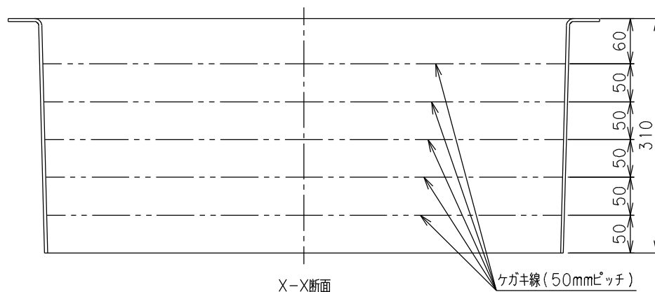
X-X断面
