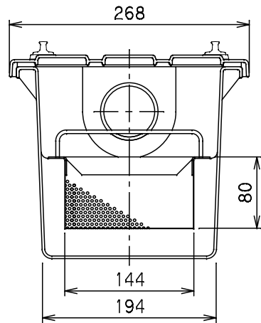
Y-Y断面図
