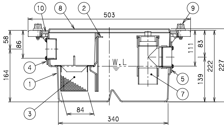
X-X断面図
