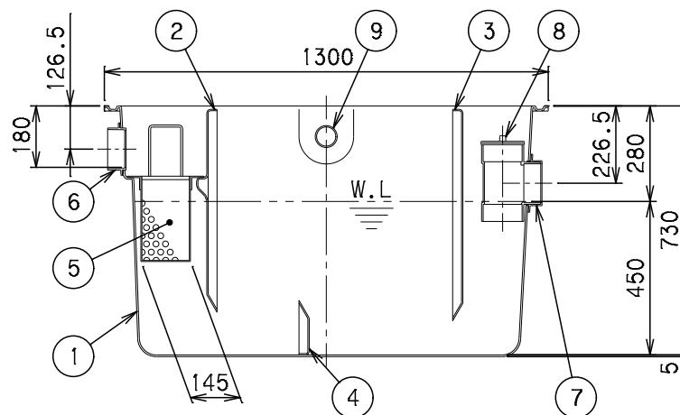
X-X断面図
