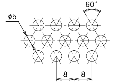
パンチングプレート打抜穴詳細
