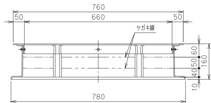
X-X断面
