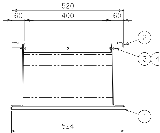
Y-Y断面
