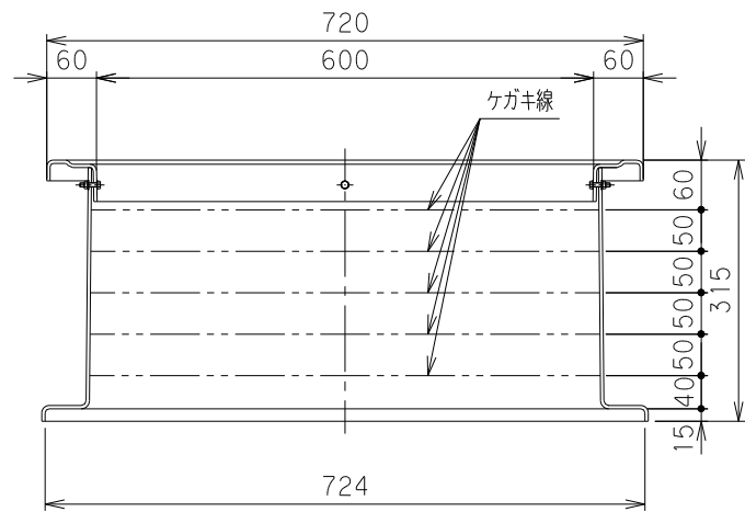
X-X断面
