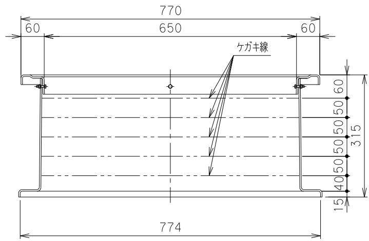
X-X断面
