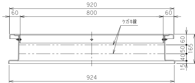
X-X断面
