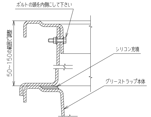
施工時詳細図
