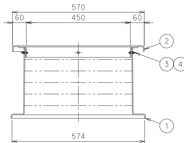
Y-Y断面
