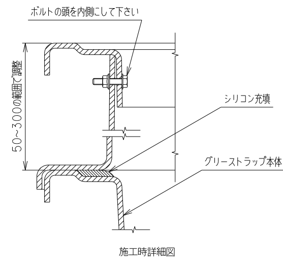
施工時詳細図
