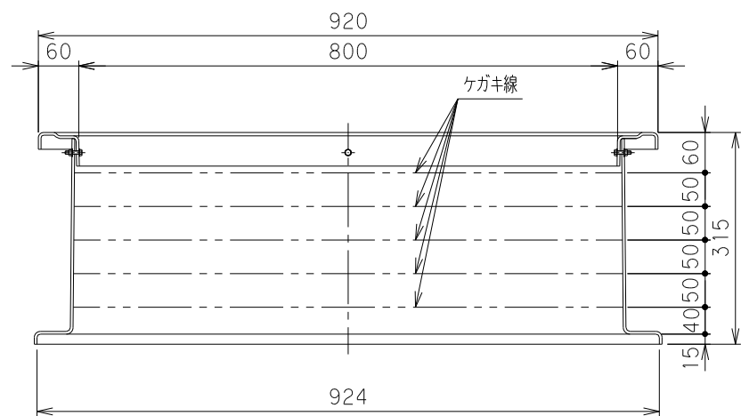
X-X断面
