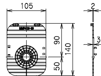
⑦ 土留板
