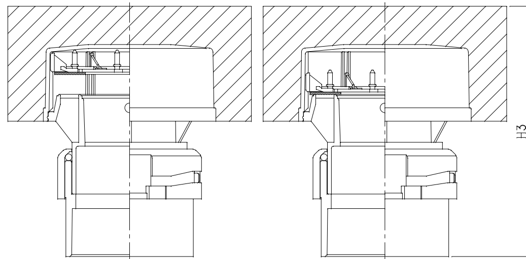
組立図 (開時)
