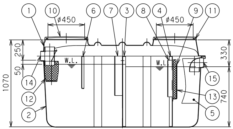
X-X断面
