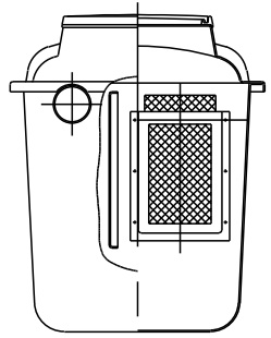
O-Z断面
