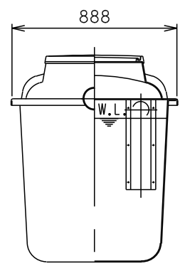
O-Y断面
