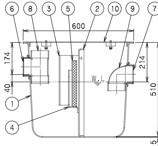
X-X断面
