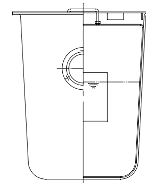
0-Z断面
