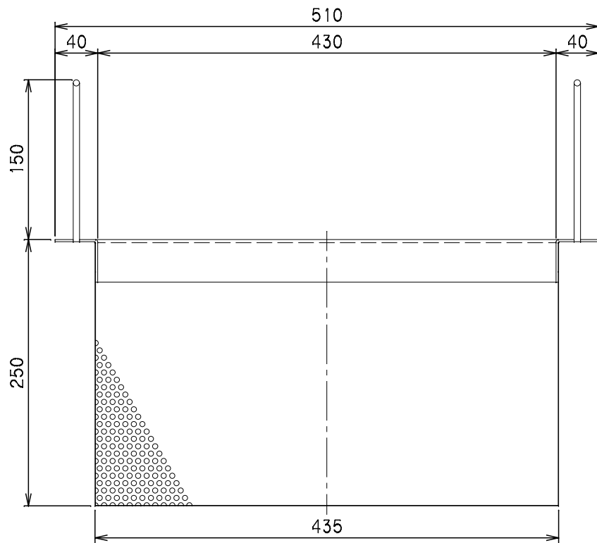
X-X断面
