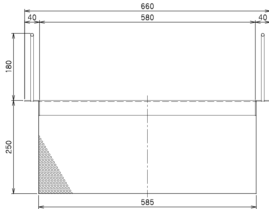
X-X断面
