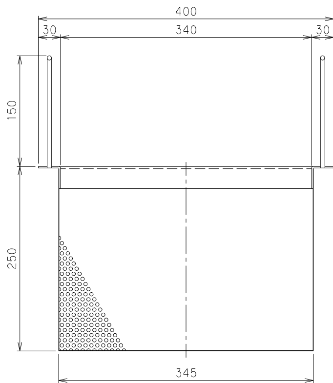
X-X断面
