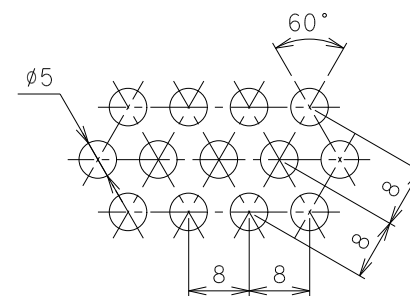
パンチングプレート打抜穴詳細
