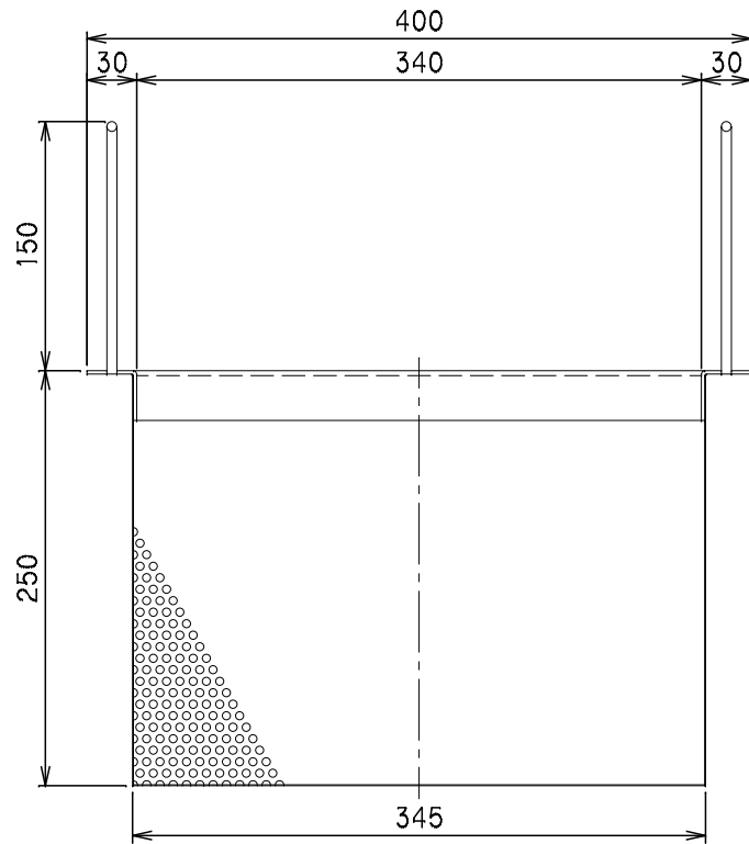
X-X断面
