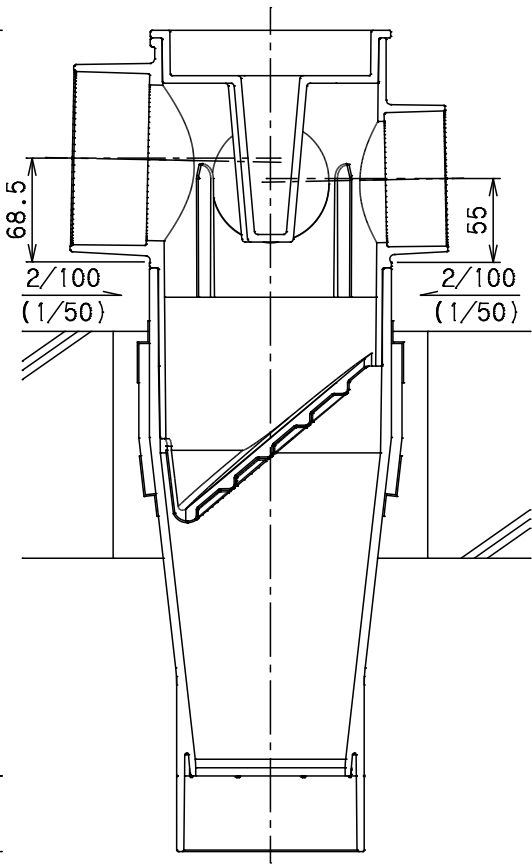
A-A' 断面図
