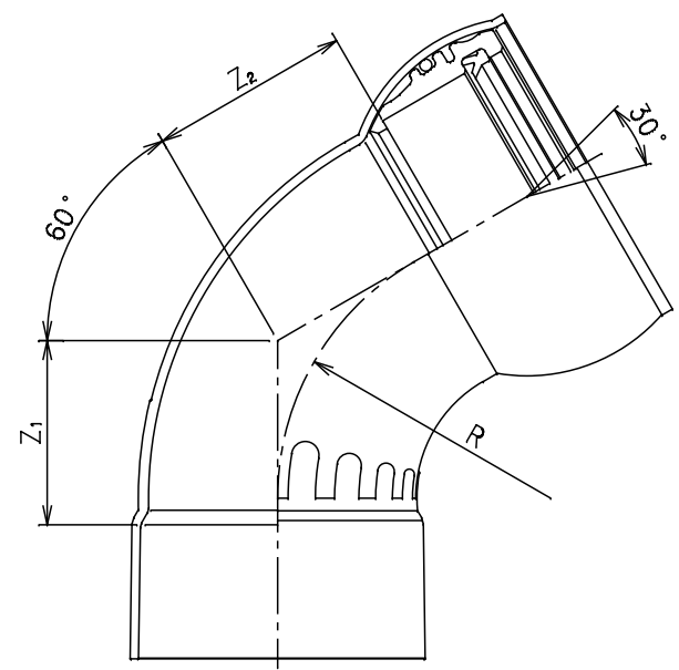
二次成形品
