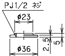
送り座 (同梱品)
