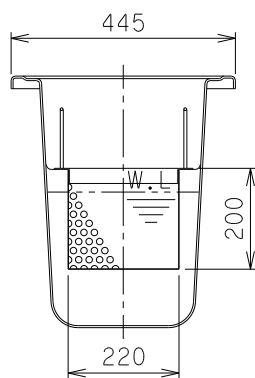
Y-Y断面図
