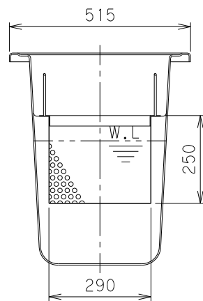
Y-Y断面図
