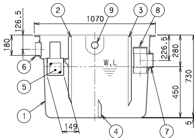
X-X断面図
