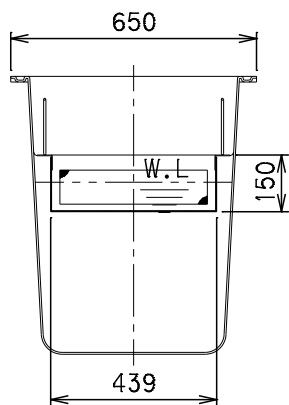
Y-Y断面図
