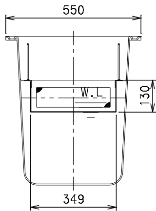
Y-Y断面図
