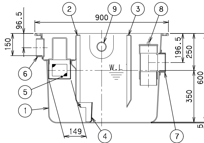
X-X断面図
