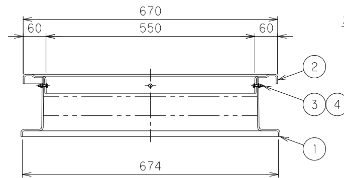
Y-Y断面
