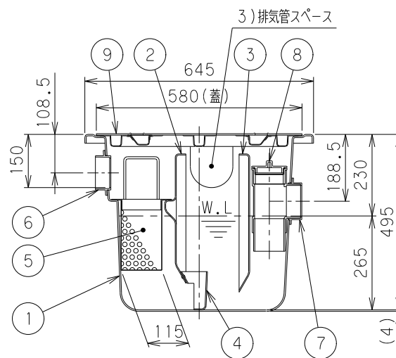
X-X断面図
