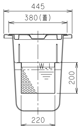
Y-Y断面図
