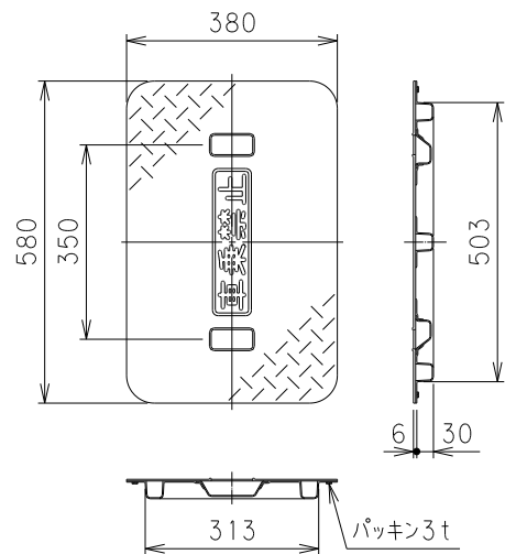
FRP蓋
