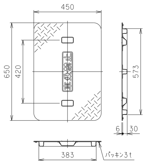
FRP蓋
