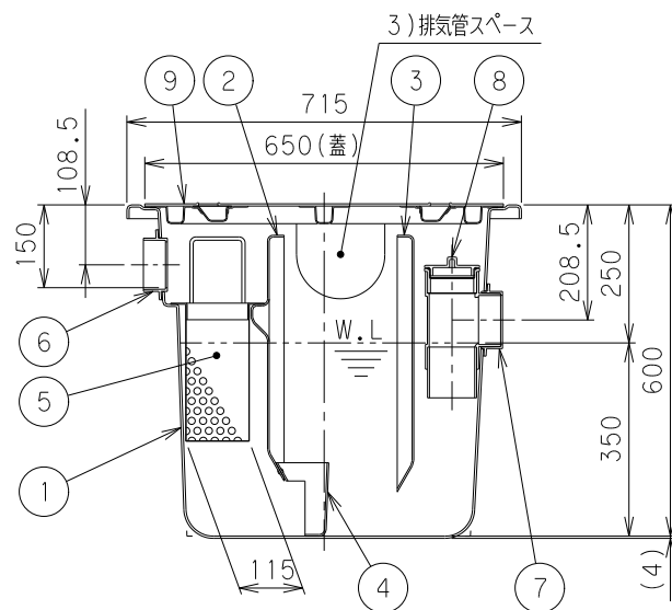
X-X断面図
