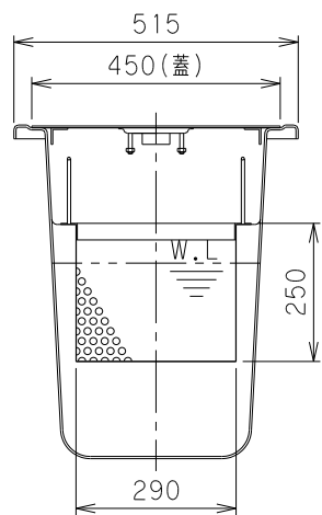
Y-Y断面図
