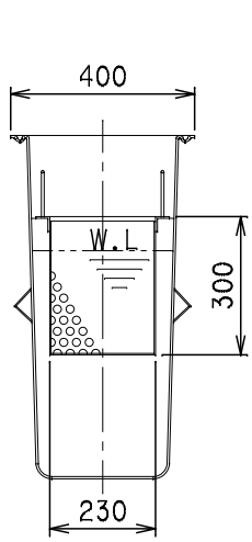
Y-Y断面図
