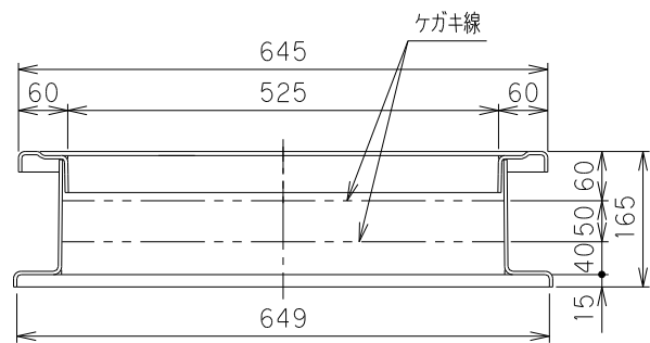
X-X断面
