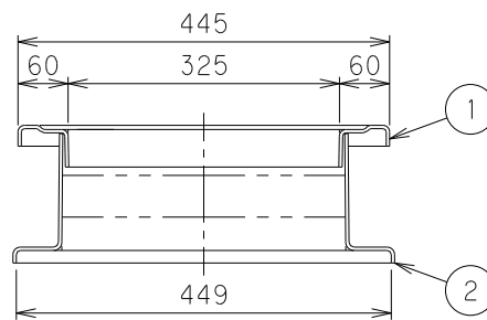
Y-Y断面
