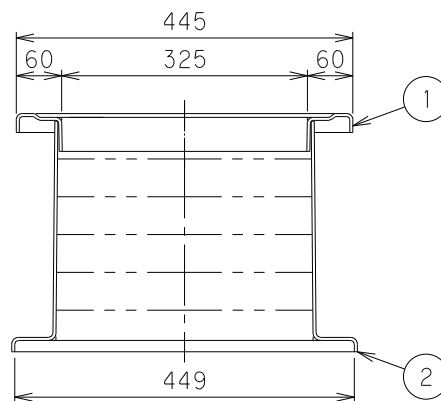
Y-Y断面
