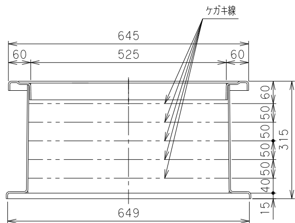
X-X断面
