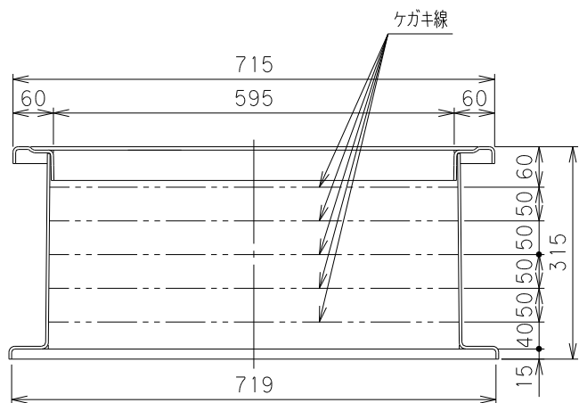
X-X断面
