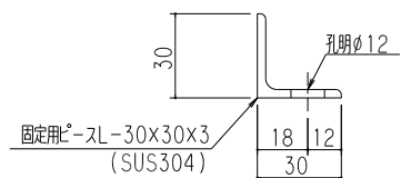
固定用ピース詳細
