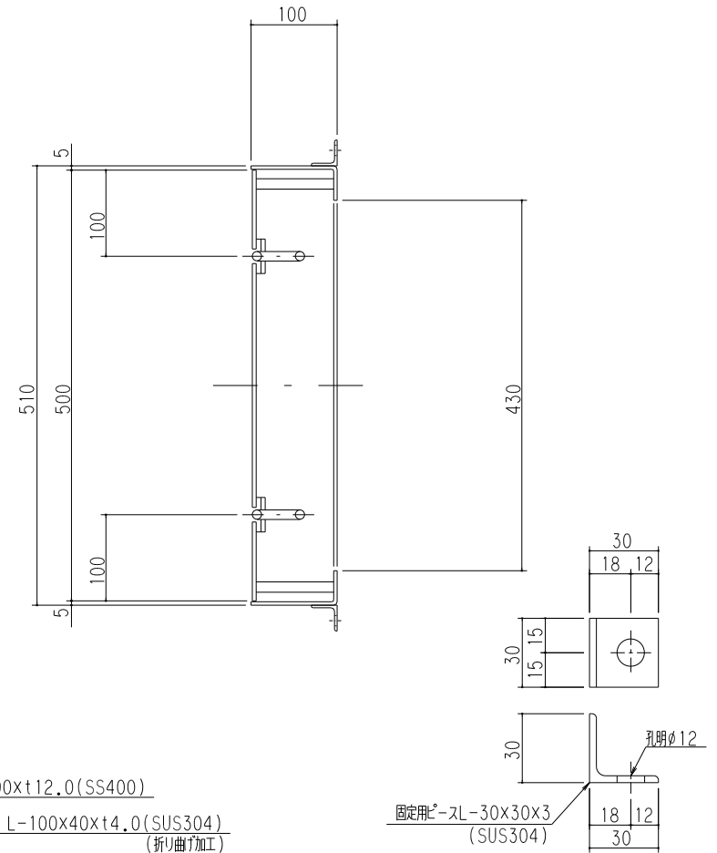
固定用ピース詳細
