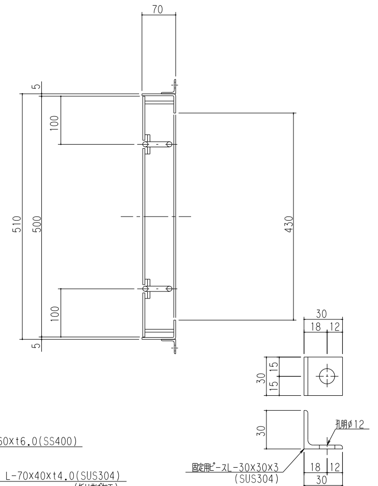
固定用ピース詳細
