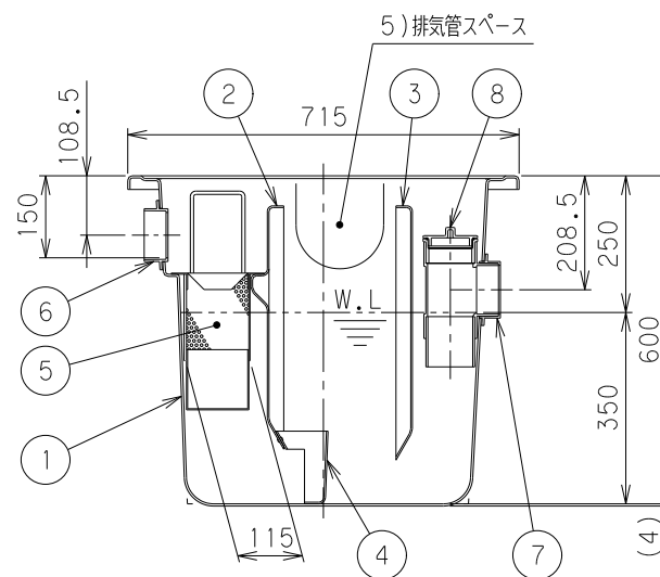
X-X断面図
