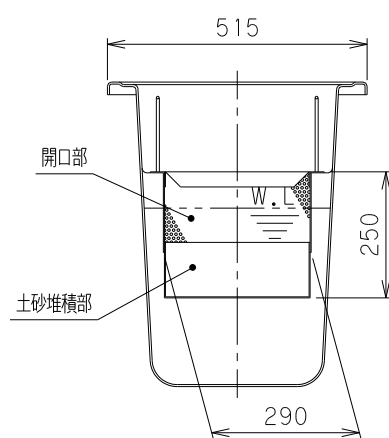
Y-Y断面図
