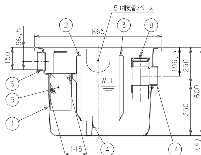
X-X断面図
