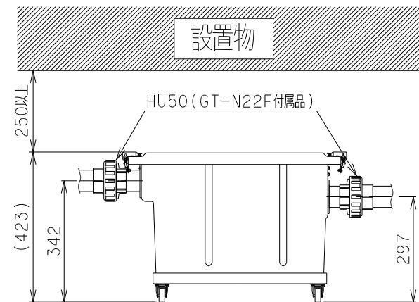
設 置 例
