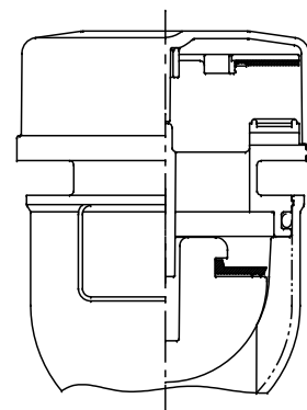
組立図(開時)
