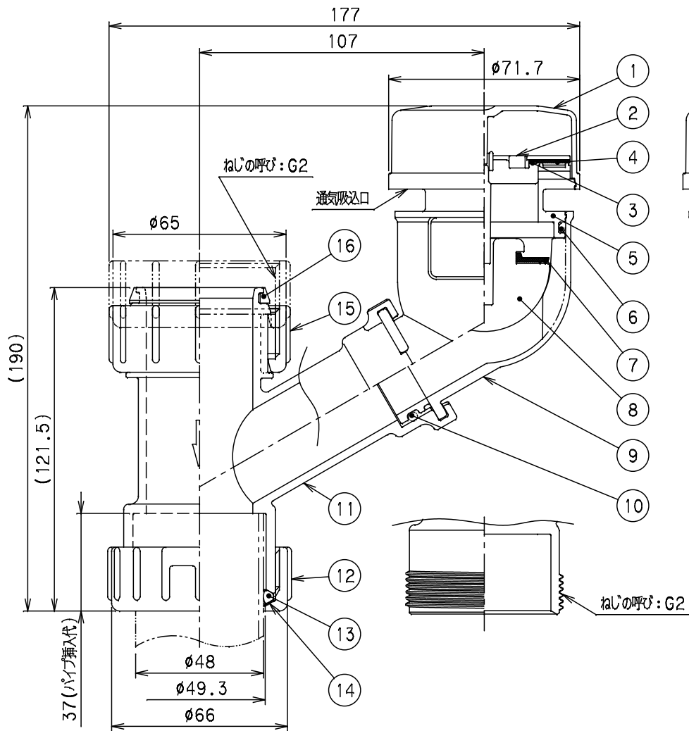
組立図(閉時)
