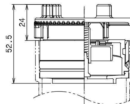
組立図 (閉時)
