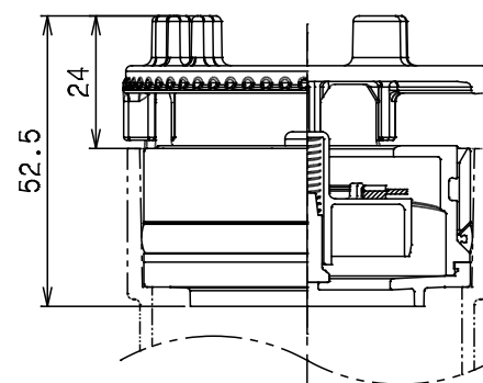
組立図 (開時)
