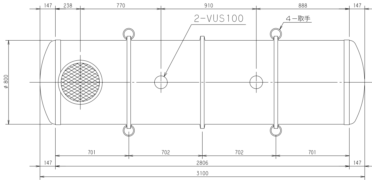
平面図
