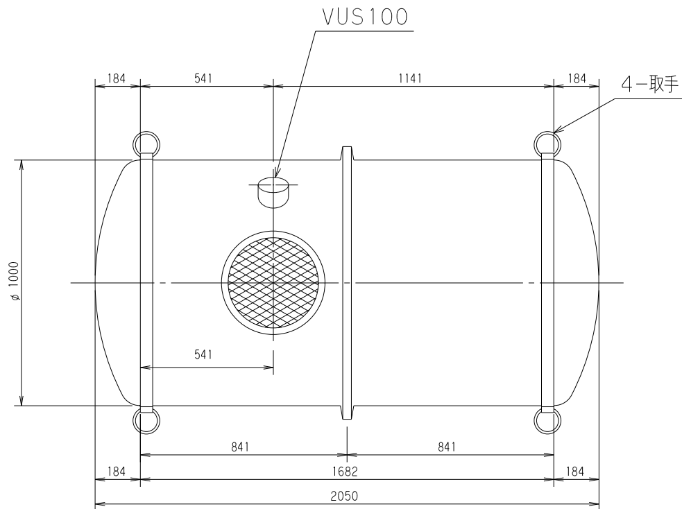
平面図
