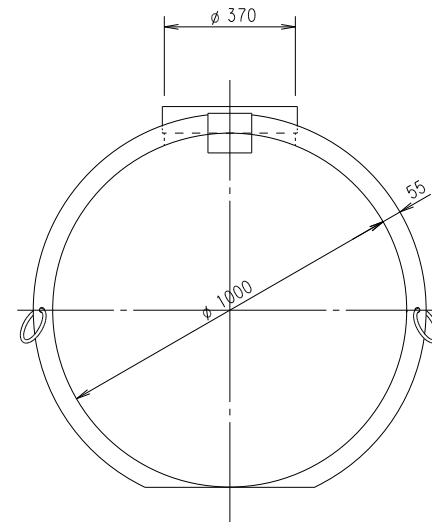
断面図
