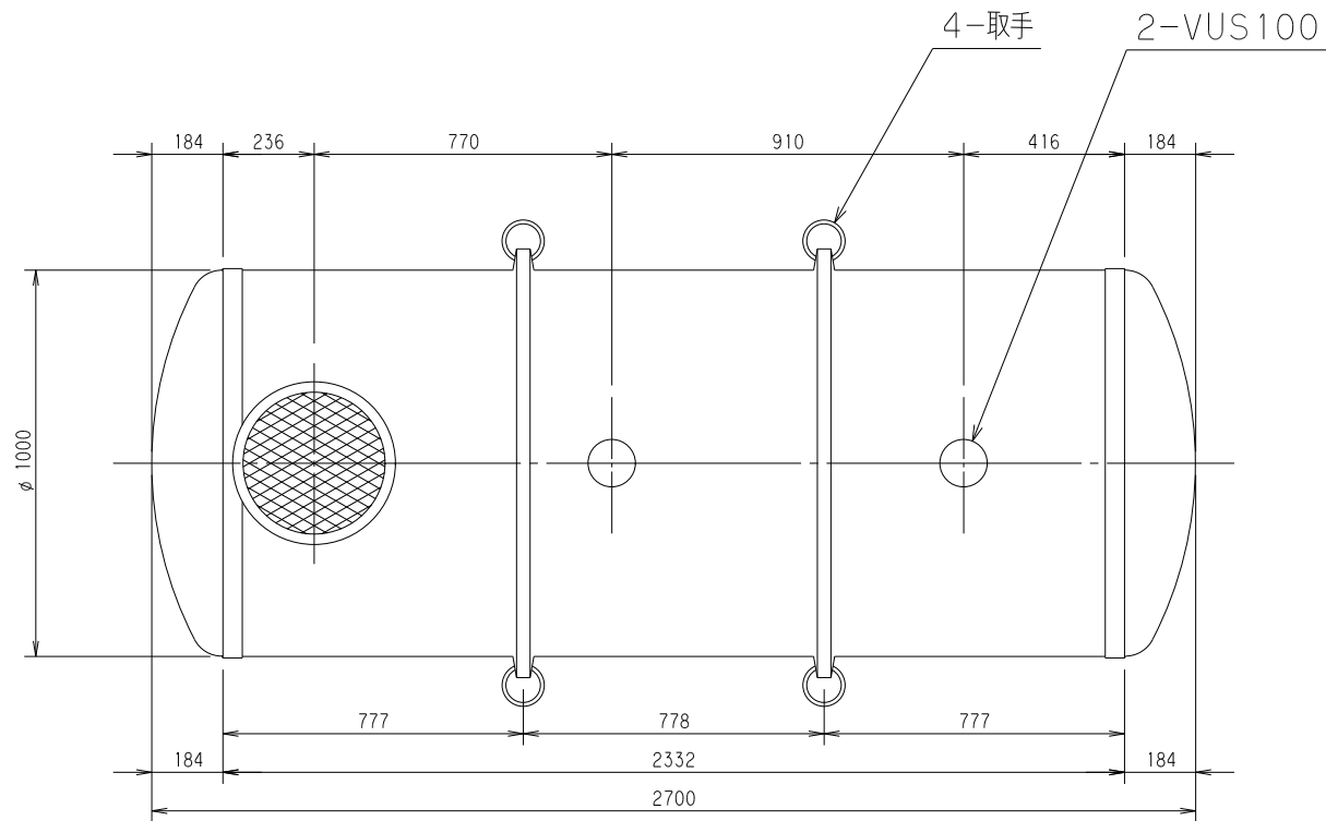
平面図
