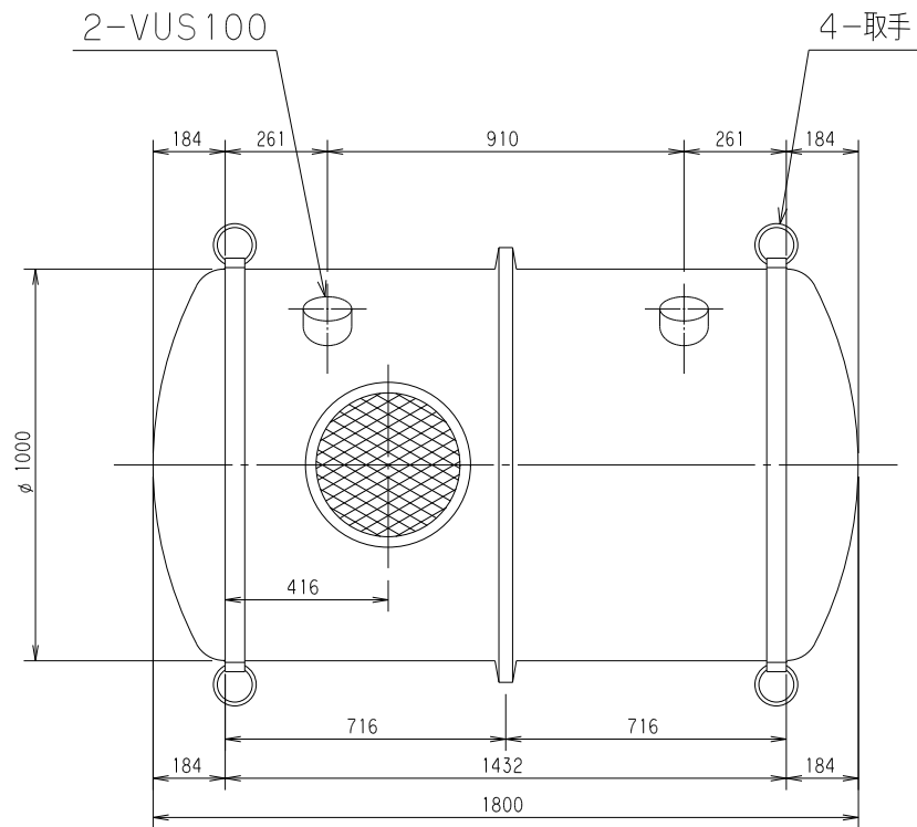
平面図
