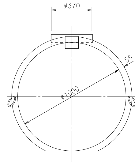
断面図
